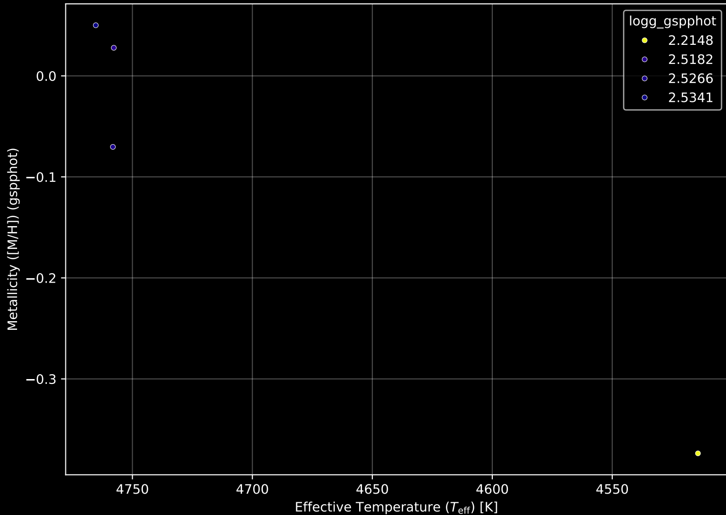
APOGEE DR17 Field: [ruprecht147] Stellar Population Parameters (n= 4)
